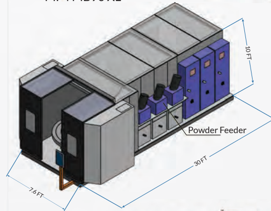
MF4 MB90 XL
